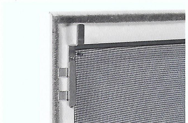
Spannrahmen mit Einhängehaken und Bürsten 5 mm
